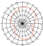
H-Plane at 2.45 GHz
